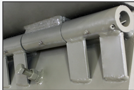
Plataforma de construcción de caja con un diseño eficiente de la plataforma y el bastidor.
