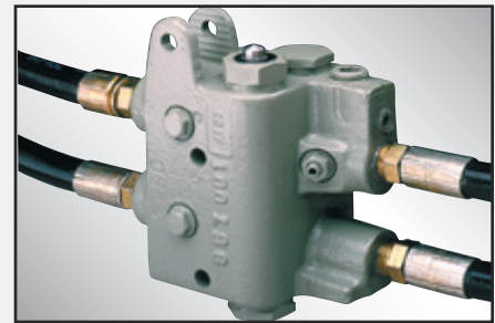
Bloque lógico de fluidos que controla el flujo del líquido hidráulico
